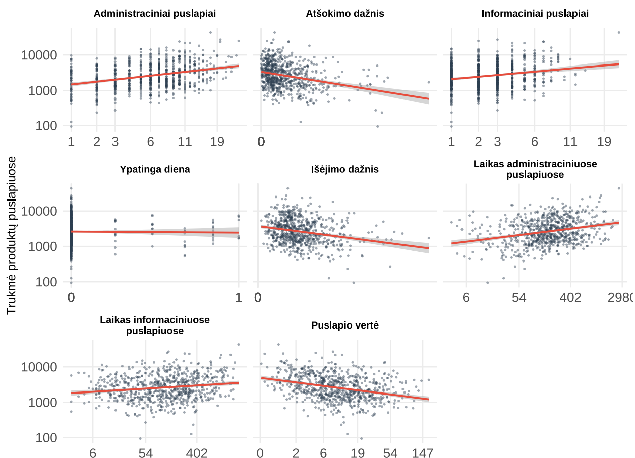
1 pav.: Sklaidos diagramos, tarp kiekybinių kovariančių ir atsako - laiko, kurį naudotojas praleidžia internetinėje parduotuvėje
